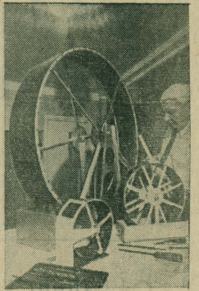
Оригинальный магнитно-тепловой двигатель роторного типа разработал московский изобретатель А. Г. Пресняков — победитель Всесоюзного конкурса на солнечный водоподъемник.
