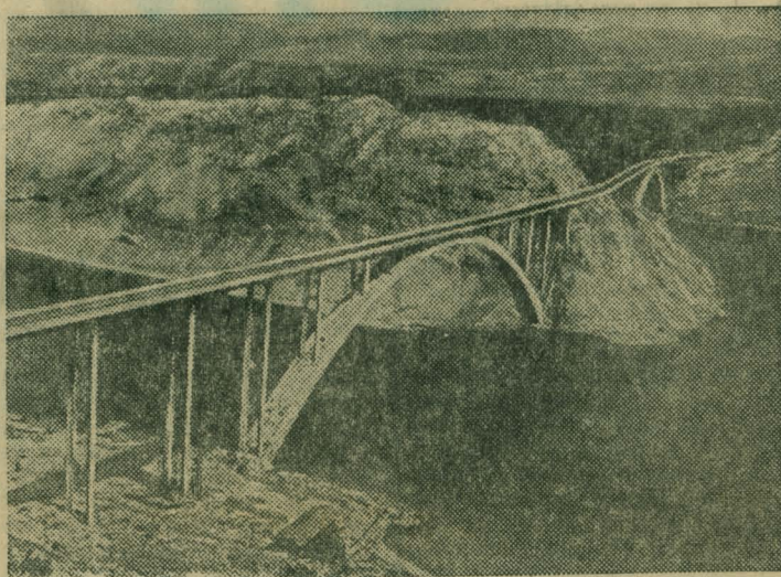
ЮГОСЛАВИЯ. Открылось регулярное автомобильное движение по новому мосту (на снимке), связавшему один из крупнейших адриатических островов Крк с материком. Длина нового двухпролетного арочного моста 1440 метров. Его огромные пролеты покоятся всего на трех опорах, в качестве промежуточной использован небольшой островок, расположенный между Кркком и берегом. Мост не мешает судоходству — под его арками свободно проходит суда. Фотохроника ТАСС.
