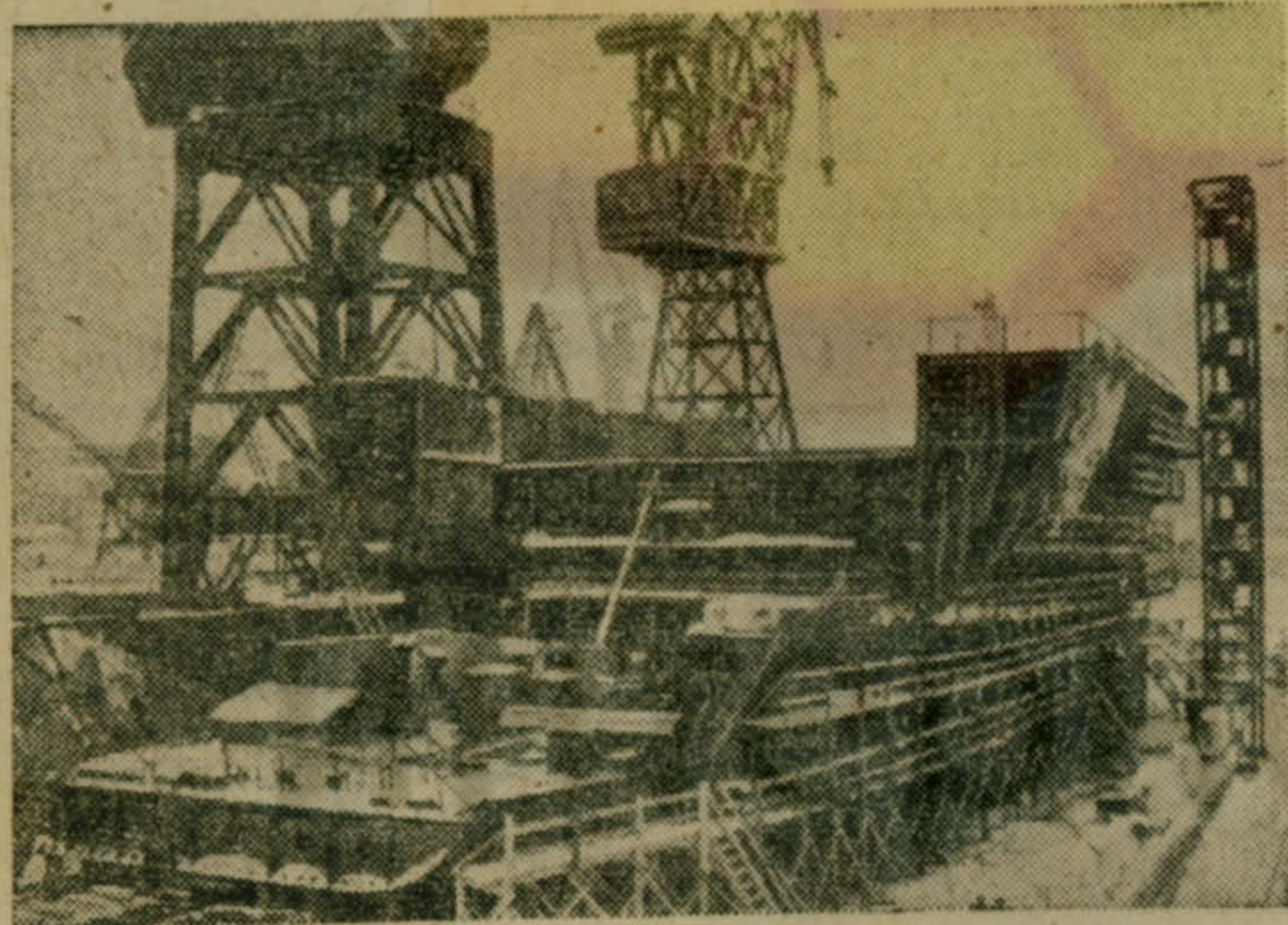
ЛЕНИНГРАД. На стапеле Балтийского завода имени С. Орджоникидзе все более рельефно просматриваются контуры очередного советского атомного ледокола «Россия» (на снимке).
