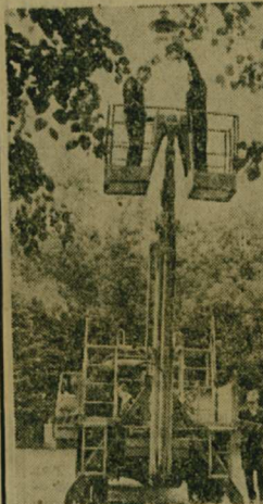
МОСКВА. Коллективом НИИглавмосавтогидротранс разработана конструкция новой телескопической вышки ТВ-3М с высотой подъема 13 метров. Изготовлена она на автомобильном заводе № 6.
