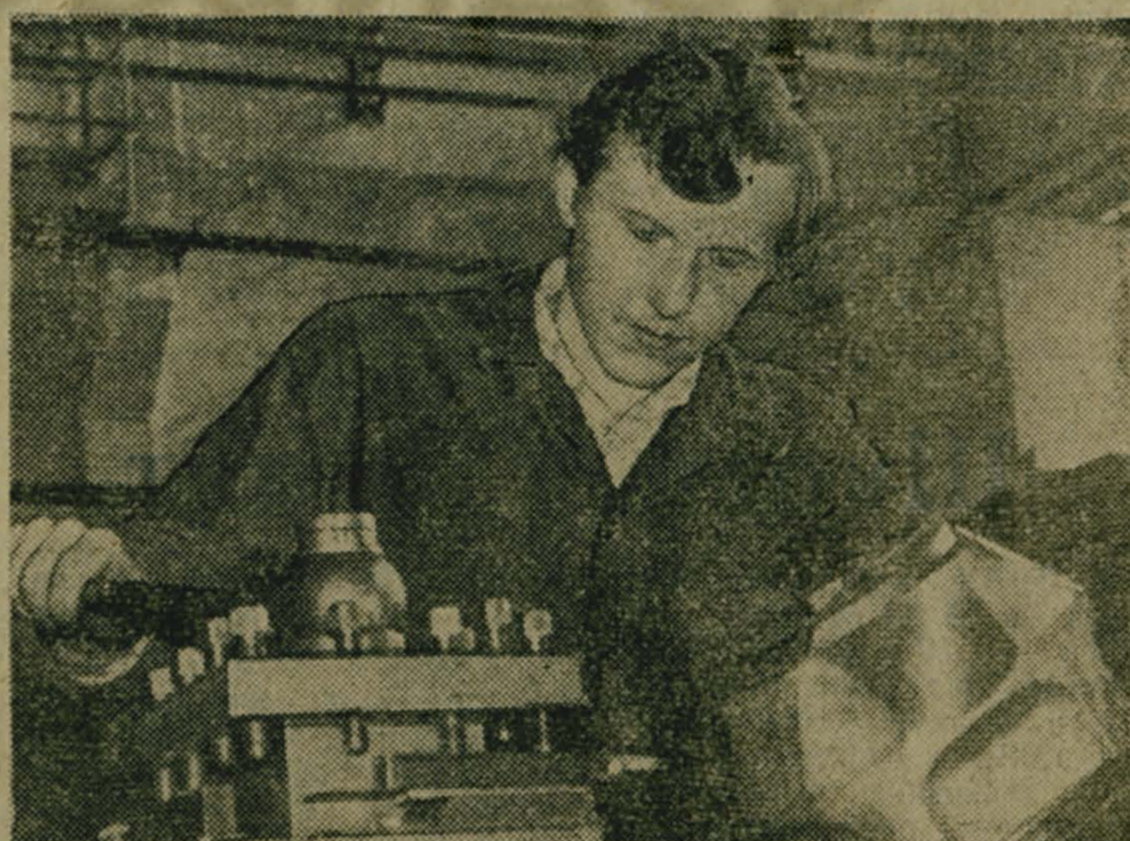
Высоким мастерством овладел токарь механического цеха экспериментального завода института буровой техники Сергей Васильевич Ермаков. Именно поэтому он участвует в изготовлении ответственных деталей для бурильного инструмента, выпускаемого заводом для нефтяников страны. Ежедневно перевыполняет задания стало правилом молодого токаря. А через его руки проходят такие детали, как расширители, корпуса, валы турбобуров. Обработка их требует точности, высокого качества. И Сергей Ермаков успешно справляется с порученным делом. В честь XXVII съезда КПСС талантливый рабочий намерен досрочно завершить личное задание года.
